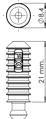
Fixi pin:
